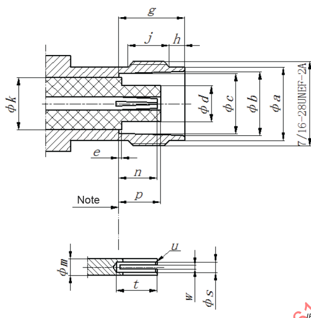
Figure 2 – Prise femelle (pour les dimensions, voir Tableau 2)
