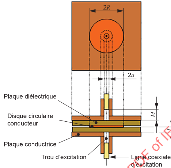
Figure 1 – Structure d'un résonateur à disque circulaire
