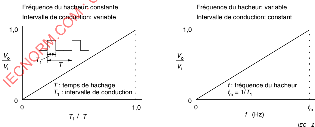
Figure 27 – Courbes caractéristiques de base de la commande d'un hacheur abaisseur
