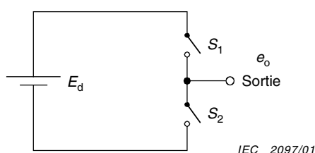
Figure 51 – Représentation caractéristique de la modulation de largeur d'impulsions
