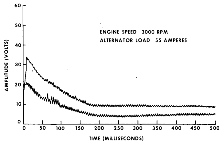
FIG. 8—LOAD DUMP TRANSIENT
